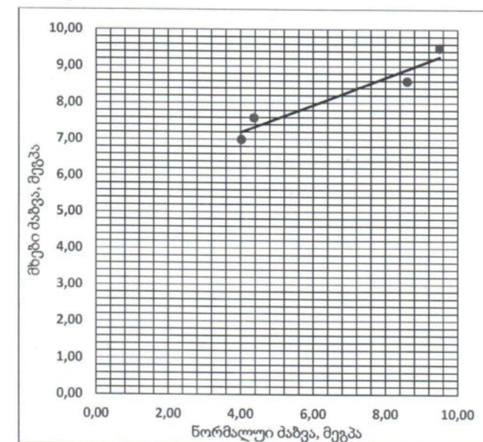
ნახ. 1 ქანის ნიმუშების ძეხვ და ნორმალურ ძაბვებს შორის დამოკიდებულების გრაფიკი. სინჯი 1.
