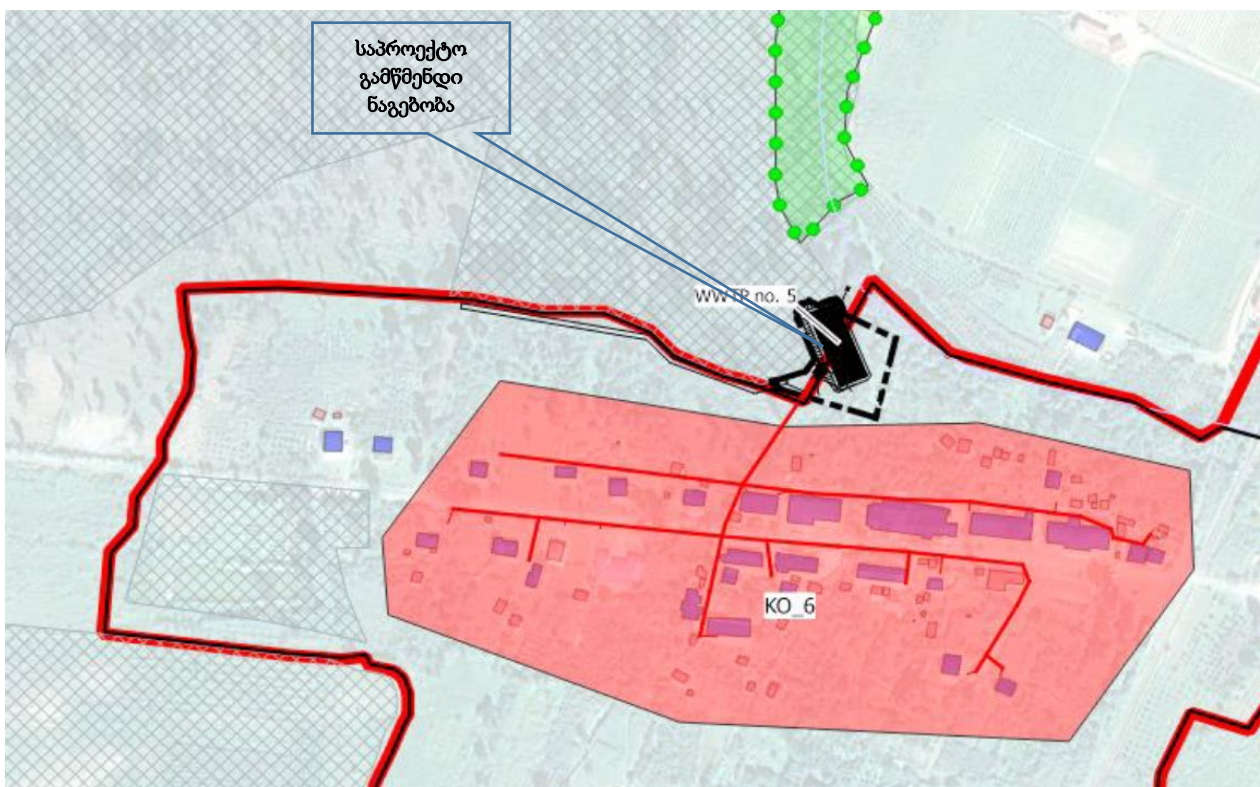
ნახაზი 3.6.1. საპროექტო საკანალიზაციო ქსელის არეალი (მონიშნულია ვარდისფრად)
